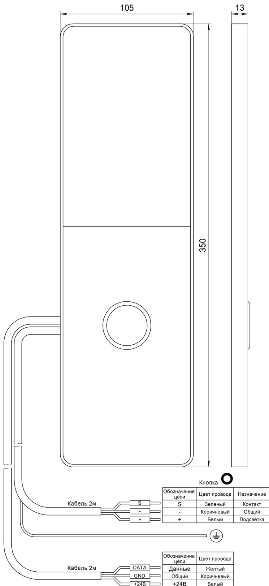
Рис.1 Внешний вид, габаритные и установочные размеры Вызывного поста МАЛАХИТ НШЕК.468381.126
